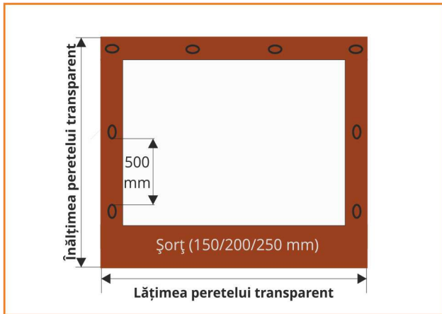
Fig. 1 - Un singur perete
