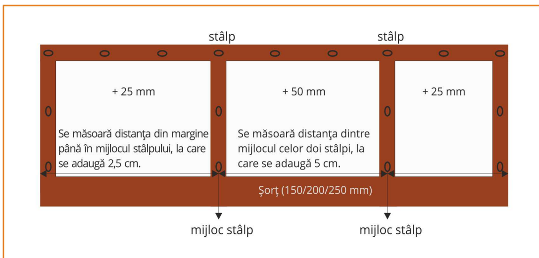
Fig. 2 - Produse alăturate, cu un singur rând de bride
